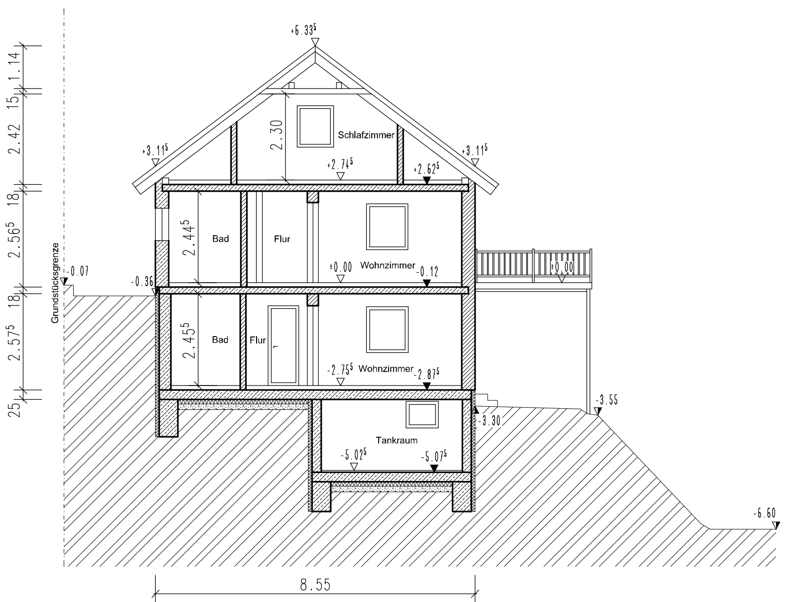
Schnitt A-A
