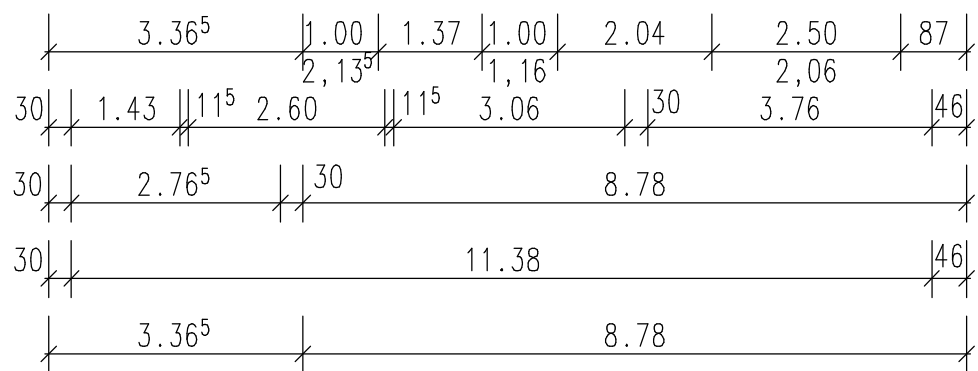
Grundriss EG
