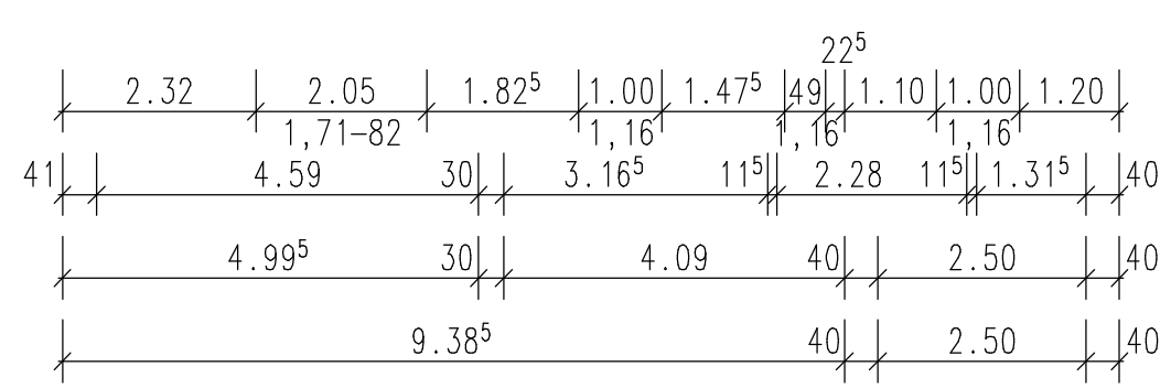
Grundriss OG
