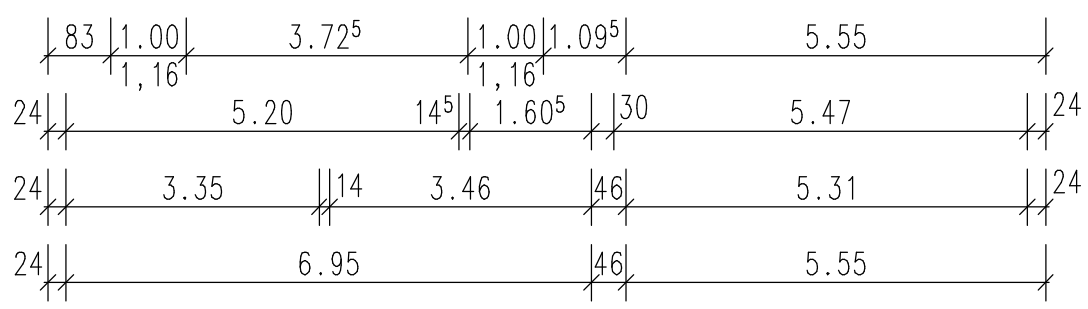
Grundriss OG
